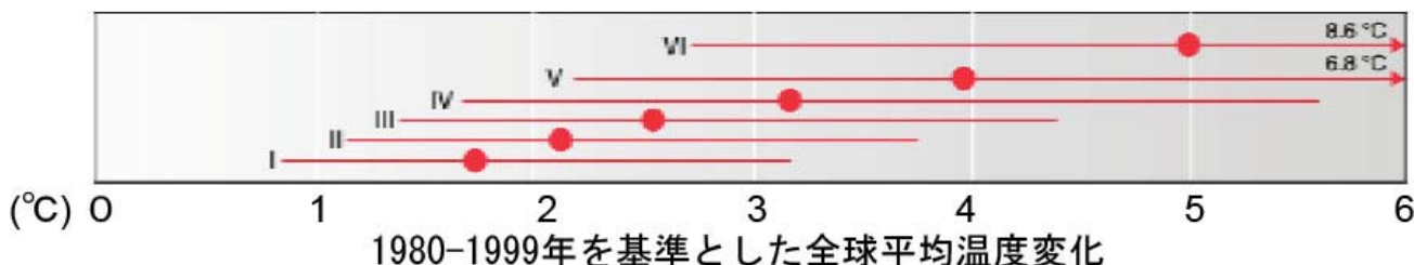
第4次評価報告書の安定化カテゴリーに対する、1980-1999年基準の予測される数世紀間の昇温の予測
