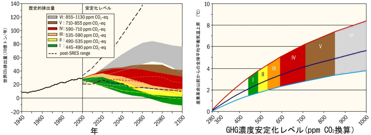
図SPM. 8. 1940年から2000年の世界のCO 2 排出量と、2000年から2100年に関する安定化シナリオカテゴリーのそれぞれに応じた排出量の範囲（左図）及び、安定化目標と産業革命以前からの可能性の高い平衡状態の世界平均気温上昇量との関係（右図）。平衡状態に至るには数世紀かかるとみられ、高い安定化レベルのシナリオについては特にその傾向が顕著である。彩色された領域は、それぞれの目標（安定化カテゴリーIからVI）に対応して分類された安定化シナリオを示す。右の図は、産業革命以前からの世界平均気温上昇の幅を示し、次のものを用いた：(i) 気候感度として「最良の見積もり」の3°C（彩色された領域の中心にある黒い線）、(ii) 気候感度として可能性が高い予測幅の上限である4.5°C（彩色された領域の上にある赤い線）、(iii) 気候感度として可能性が高い予測幅の下限である2°C（彩色された領域の下部にある青い線）。左図の黒の破線はSRES（2000）以降に発表された最近のベースラインシナリオの排出量の幅を示す。CO 2 のみの、及び複数の温室効果ガスに関する安定化シナリオの排出量の、すべてのシナリオ分布の中の第10パーセンタイルから第90パーセンタイルの幅を示す。注）ほとんどのモデルのCO 2 排出量には、伐採及び森林減少後に残る地上バイオマスの腐食（分解）からの排出量及びピートの火事、水抜き後のピート土の腐食から生じる排出量は含まれない。[図SPM. 7, SPM 8]
